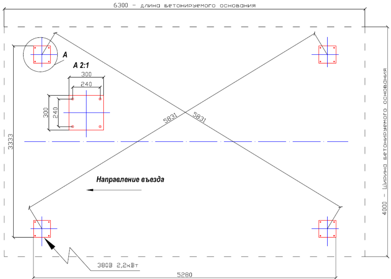
Рис. 2а. Установочные размеры подъёмника
