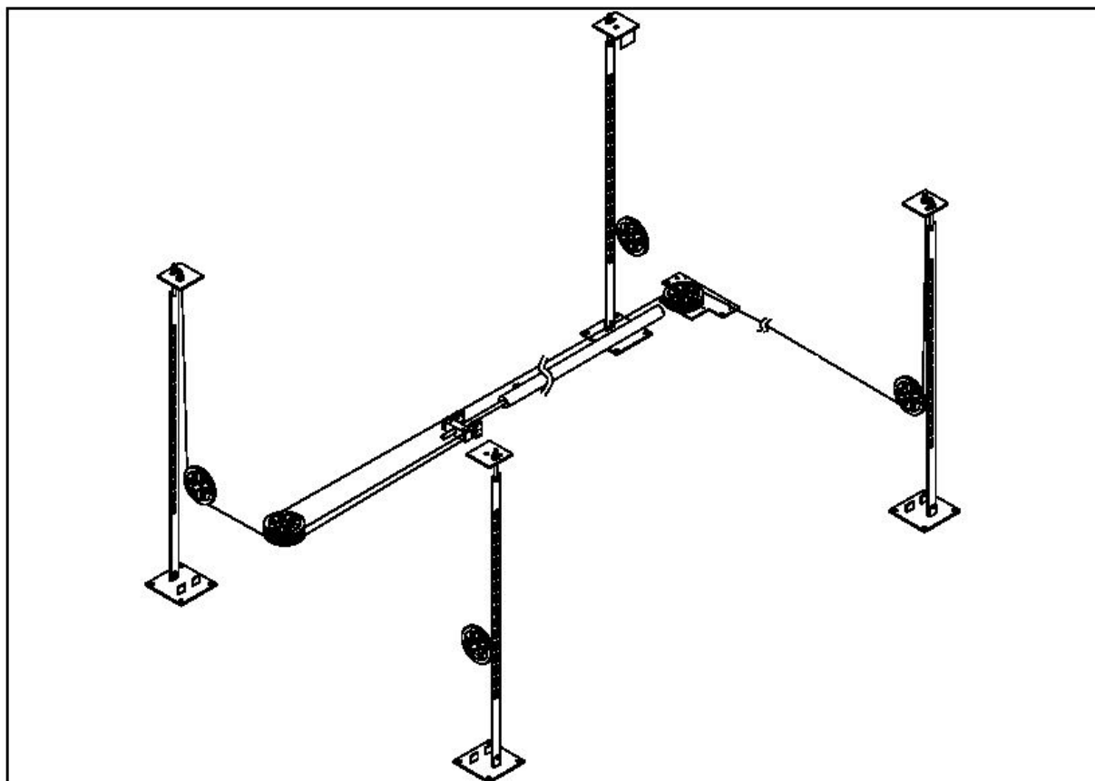
Рис. 3 (а) Схема установки и крепления тросовой системы подъёмника
