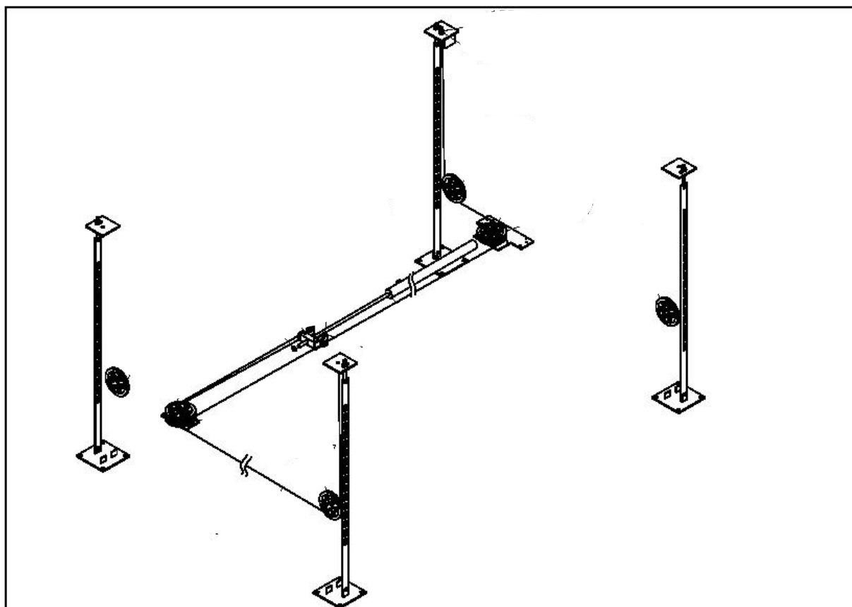
Рис. 3 (б) Схема установки и крепления тросовой системы подъёмника
